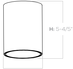
D1: 4-1/2"
